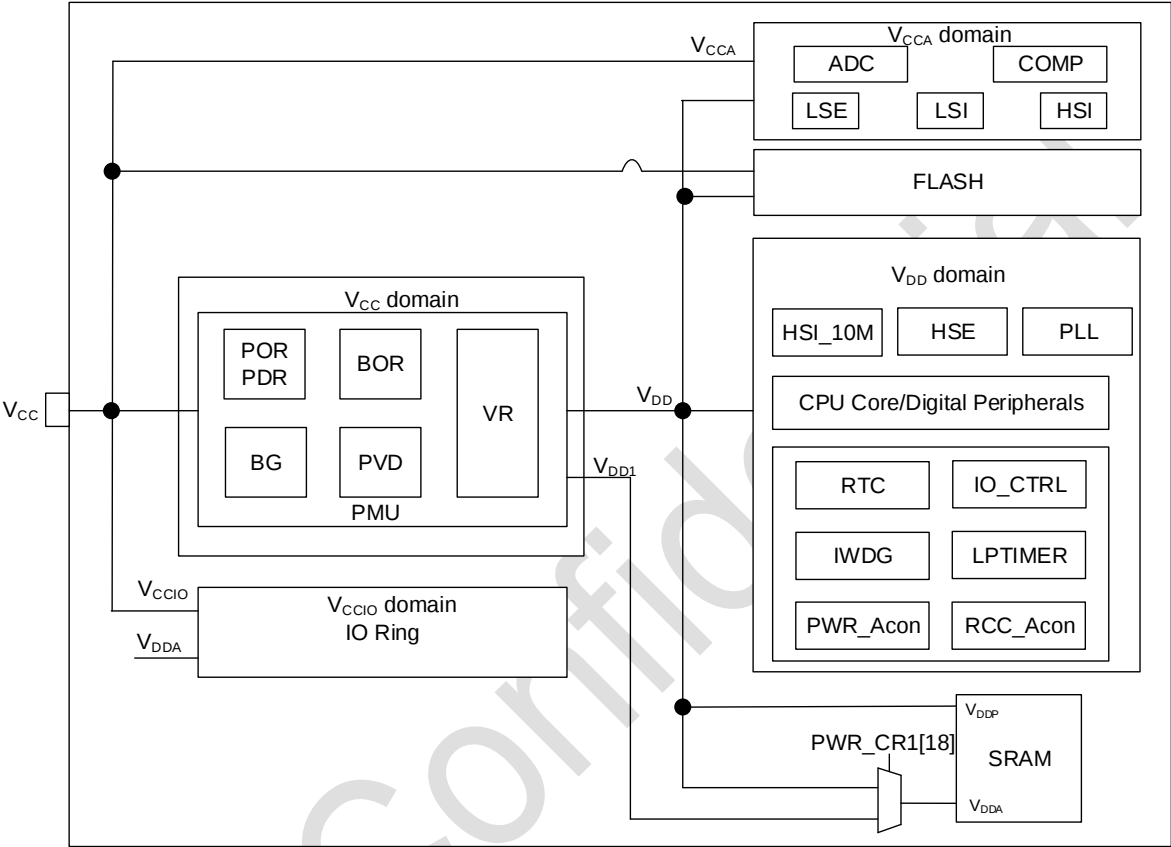
图 2-2 电源框图
