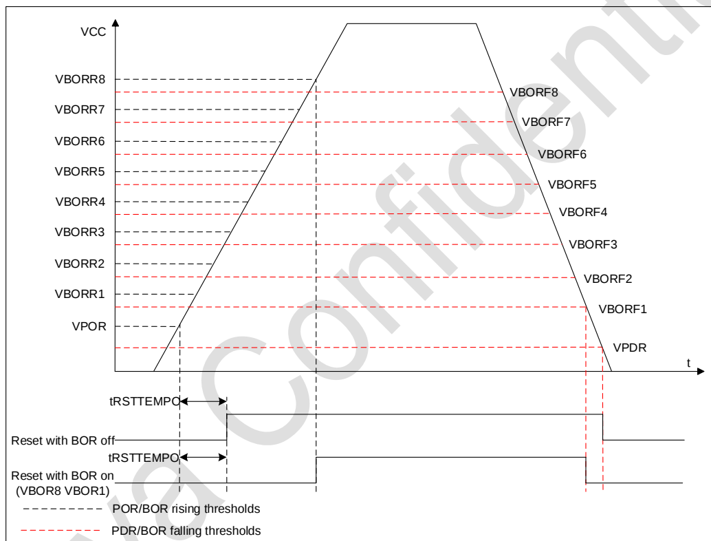
图 2-3 POR/PDR/BOR 阈值
