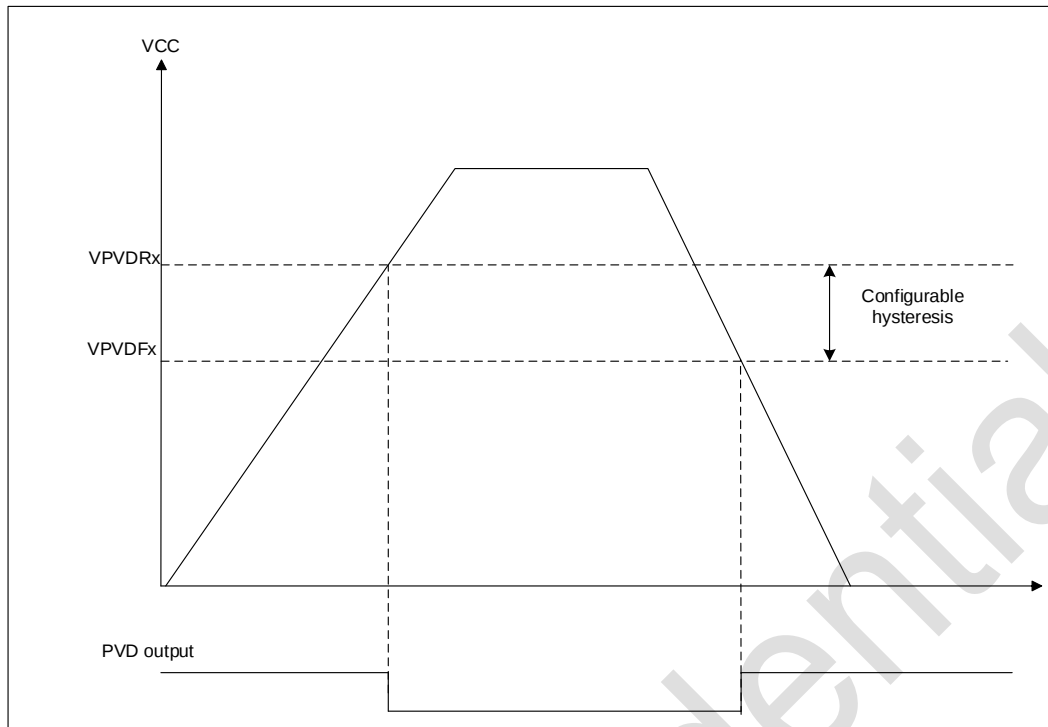
图 2-4 PVD 阈值
