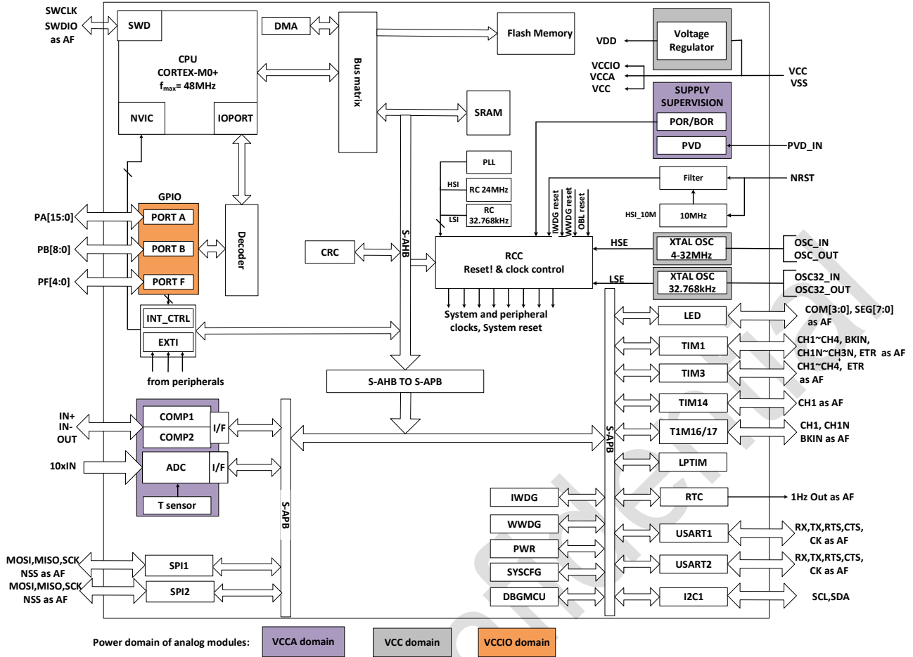
图 1-1 功能模块
